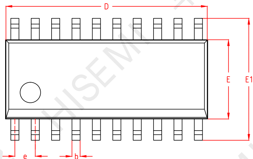
TOP VIEW 正视图
